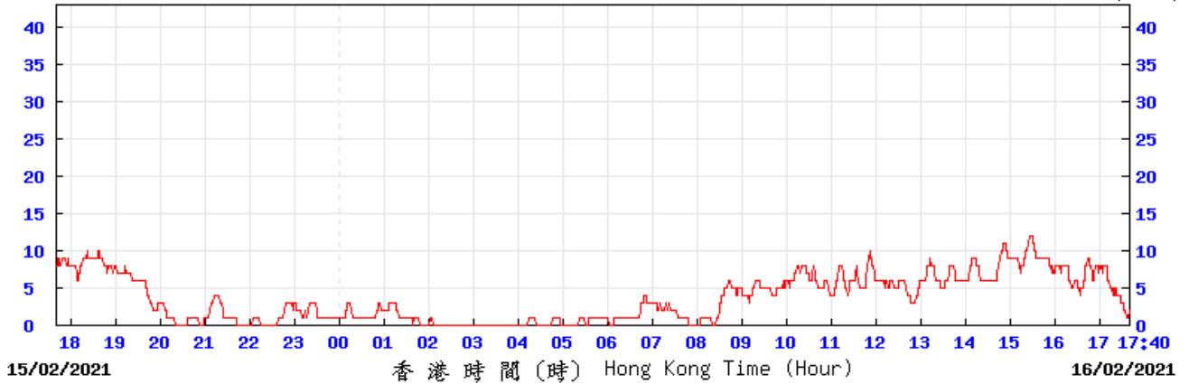
(公里/小時) (於香港時間 2021年 2月16日17時40分更新) (Updated at 17:40H on 16 Feb 2021) (km/h)
