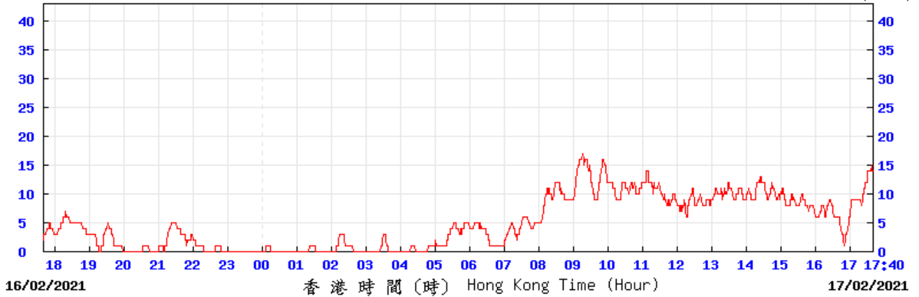
(公里/小時) (於香港時間 2021 年 2月17日17時40分更新) (Updated at 17:40H on 17 Feb 2021) (km/h)
