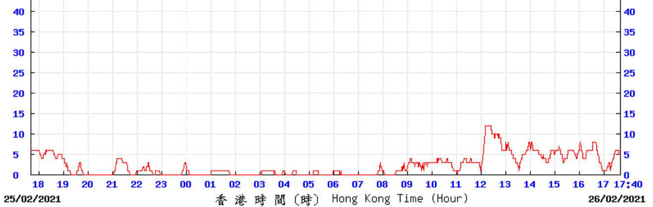
MLPC © 香港天文台 Hong Kong Observatory
