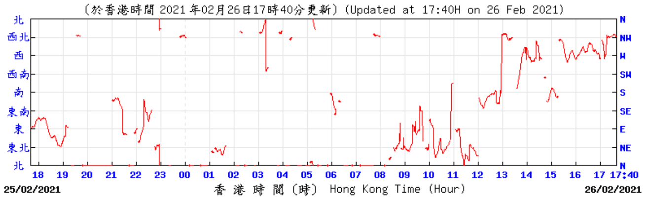
MLPC © 香港天文台 Hong Kong Observatory (公里/小時) (於香港時間 2021年 2月26日17時40分更新) (Updated at 17:40H on 26 Feb 2021) (km/h)
