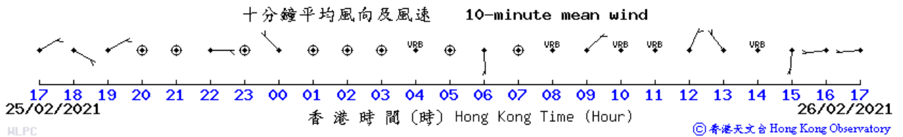
MLPC © 香港天文台 Hong Kong Observatory
