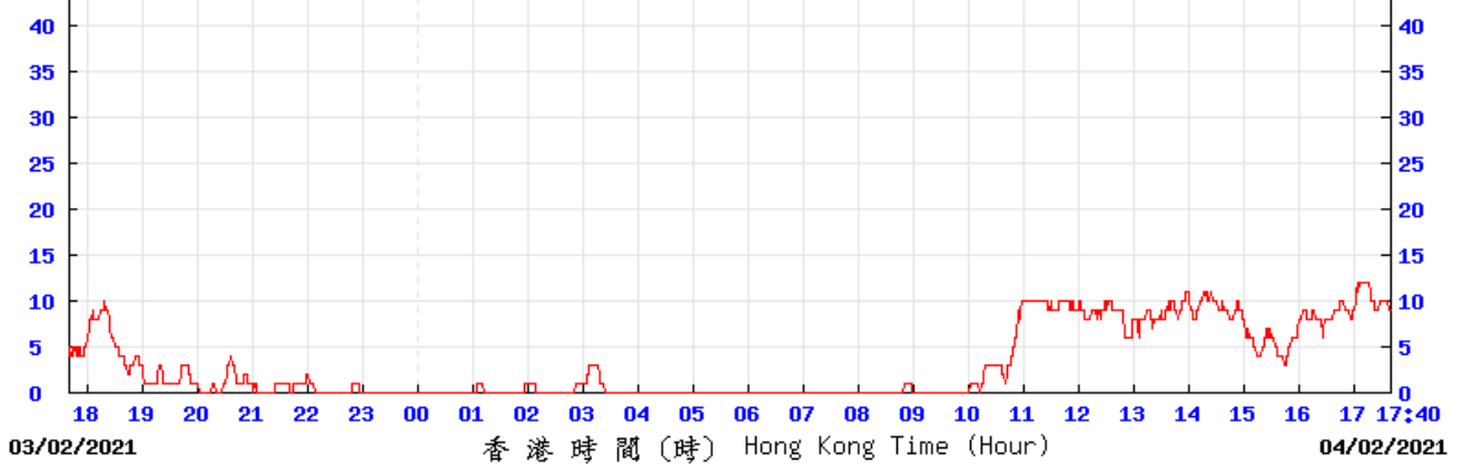
MLPC (公里/小時) (於香港時間 2021年 2月 4日17時40分更新) (Updated at 17:40H on 4 Feb 2021) (km/h)
