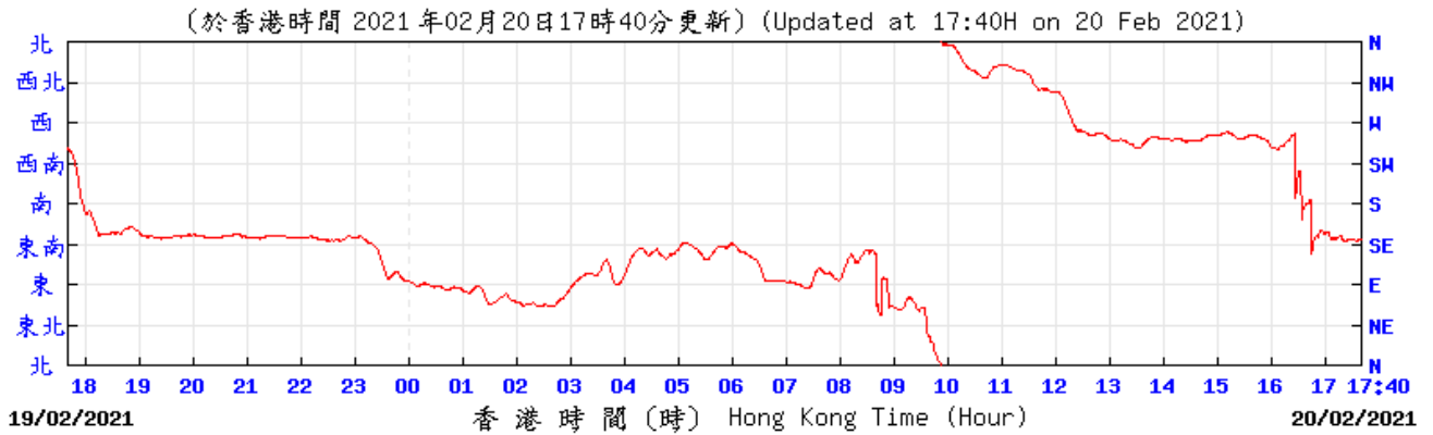
LFSC © 香港天文台 Hong Kong Observatory (公里/小時) (於香港時間 2021年 2月20日17時40分更新) (Updated at 17:40H on 20 Feb 2021) (km/h)
